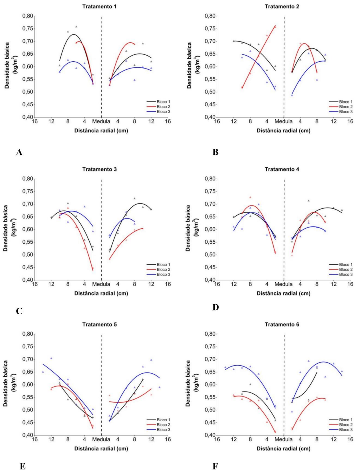
Figura 20. Efeito do espaçamento e da posição radial na densidade básica da madeira de T. vulgaris . Fonte: Autor.
