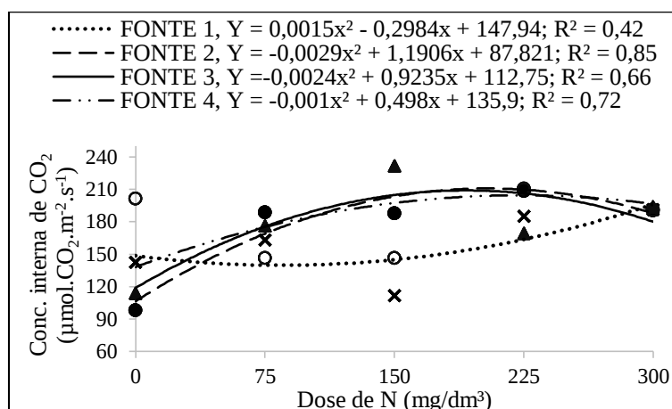
Figura 13. Concentração interna de \text{CO}_2 ( C_i ) de mudas de T. vulgaris em resposta às doses de nitrogênio, para quatro fontes testadas (FONTE 1 = ureia; FONTE 2 = sulfato de amônio; FONTE 3 = nitrato de amônio e FONTE 4 = nitrato de cálcio), ao final do experimento ( \alpha = 0,05 ).
