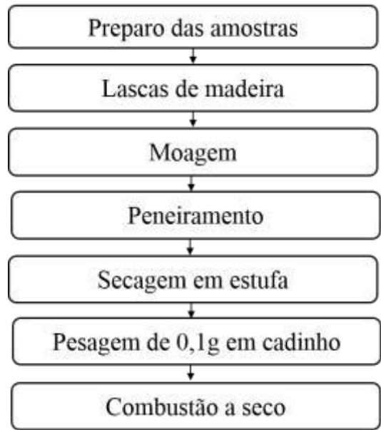
Figura 8 – Procedimento laboratorial para a determinação do teor de carbono pelo método direto.
