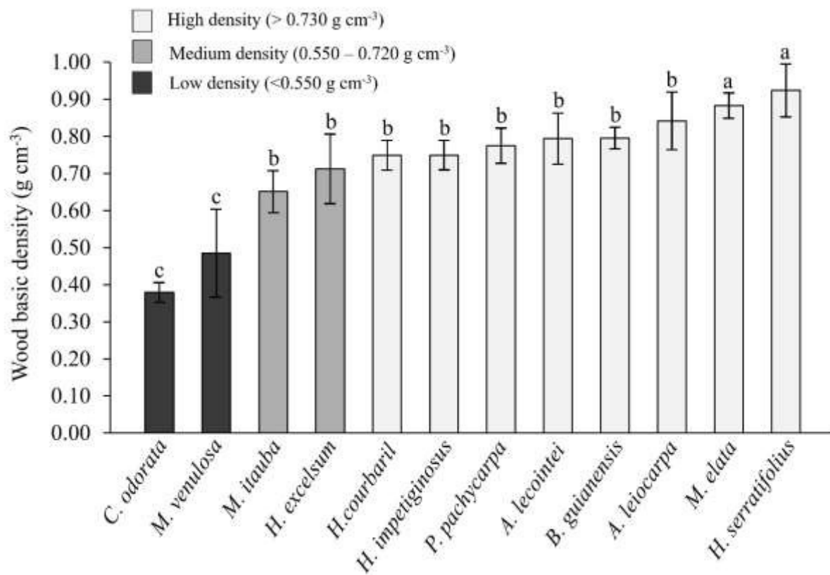
Figura 11 – Valores médios de densidade básica obtidos para a madeira das espécies em estudo.
