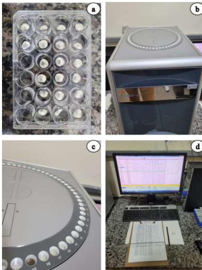
Figura 10 – Análise de teor de carbono: a) material em cadinhos; b) Equipamento para determinação do teor de carbono, analisador elemental vario PYRO cube; c) local de inserção dos cadinhos; d) computador acoplado.
